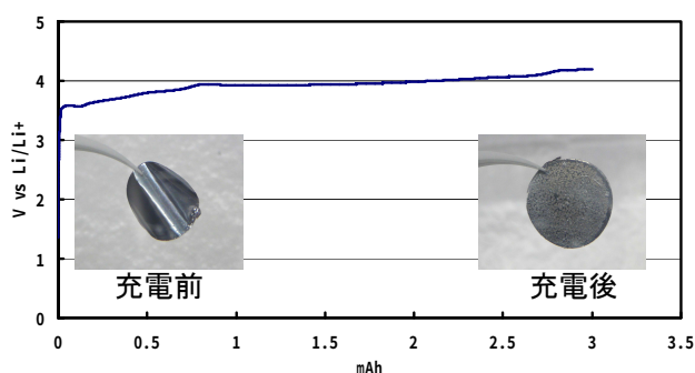
図1 充電曲線およびSi負極の形態観察
