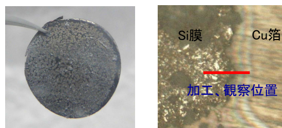
図2 充電後の形状観察結果: Si膜の変質、Cu箔の露出
