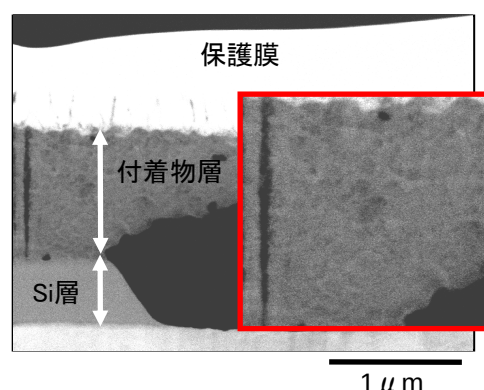
図4 冷却FIB加工+室温SEM観察
