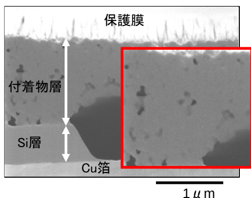
図3 冷却FIB加工+冷却SEM観察
